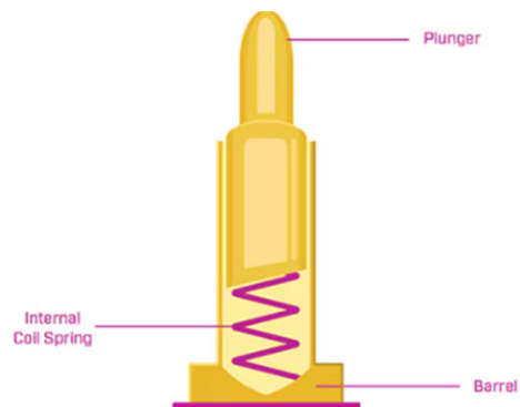
図1：代表的なポゴピンの基本部品。(画像提供：Same Sky,)
